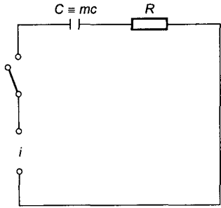
Figura 2.34 Analogía eléctrica de la figura 2.33
