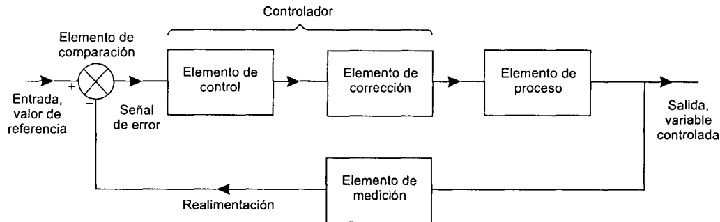
Figura 1.10 Subsistemas en un sistema de control en lazo cerrado
