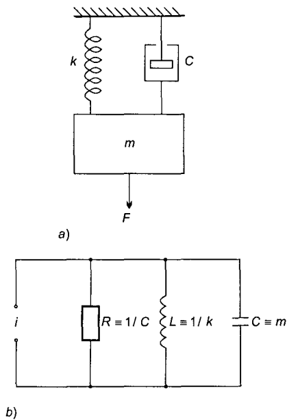
Figura 2.21 Analogías mecánica y eléctrica
