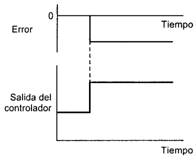
Figura 10.2 Sistema con control proporcional
