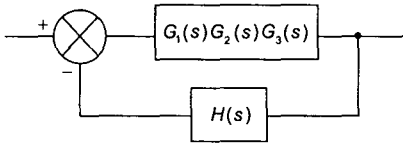
Figura 6.7 Sistema equivalente para la figura 6.6
