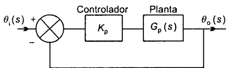
Figura 10.3 Sistema con control proporcional
