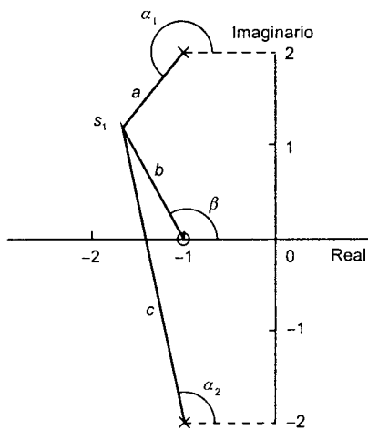
Figura 9.13 G_o(s) = K(s+1)/(s^2 + 2s + 5)
