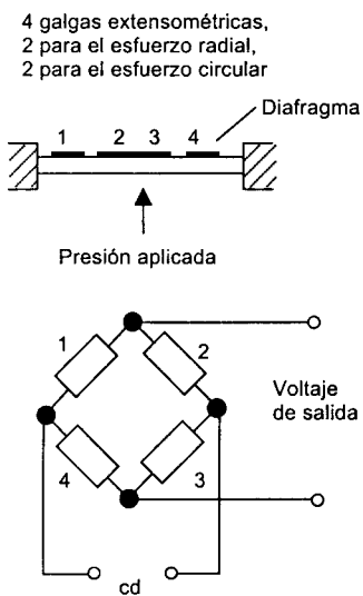
Figura 12.6 Celda de presión
